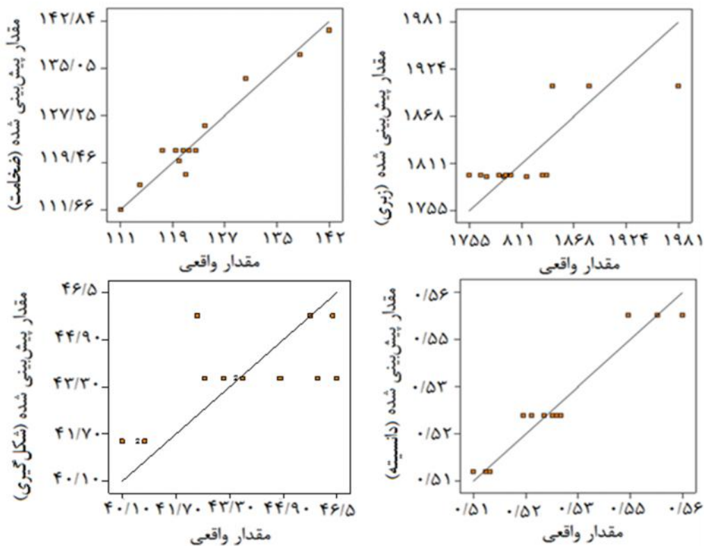
شکل ۳- نمودار پراکندگی برای خواص فیزیکی کاغذ (ضخامت، زبری، شکل گیری و دانسیته ظاهری)
