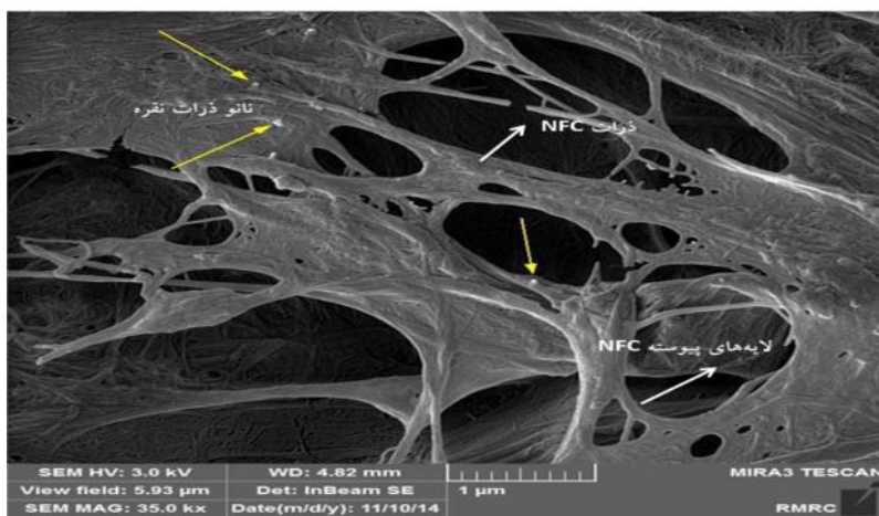
شکل ۶- تصاویر FESEM از نانو کامپوزیت NFC / نانو نقره ۱۰ ppm
