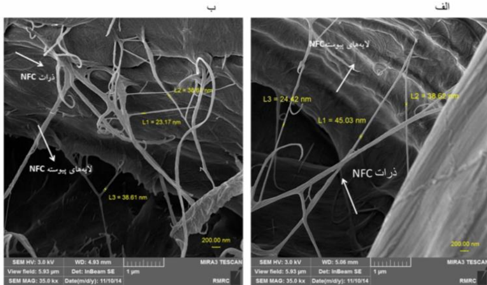
شکل ۵- تصاویر FESEM از فیلم ساخته شده با سلولز نانوفیبریله شده
