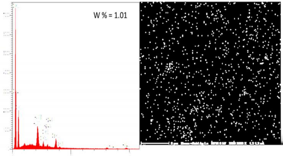
شکل ۹- (الف) MAP نانوکامپوزیت NFC/ نانونقره در سطح نقره مصرفی ۱۰ ppm و (ب) نمودار آنالیز عنصری نمونه
