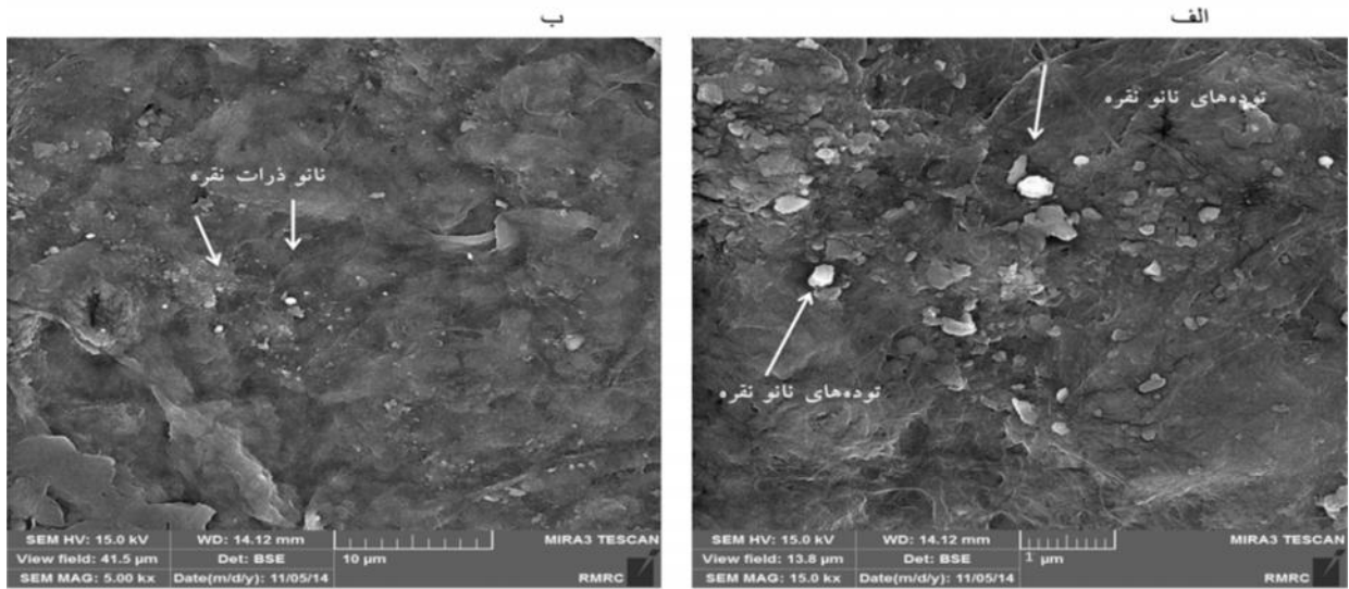
شکل ۷- تصاویر FESEM از سطح فیلم NFC تیمار شده با نانو ذرات نقره در سطح مصرفی ۱۰ ppm به روش غوطه‌وری
