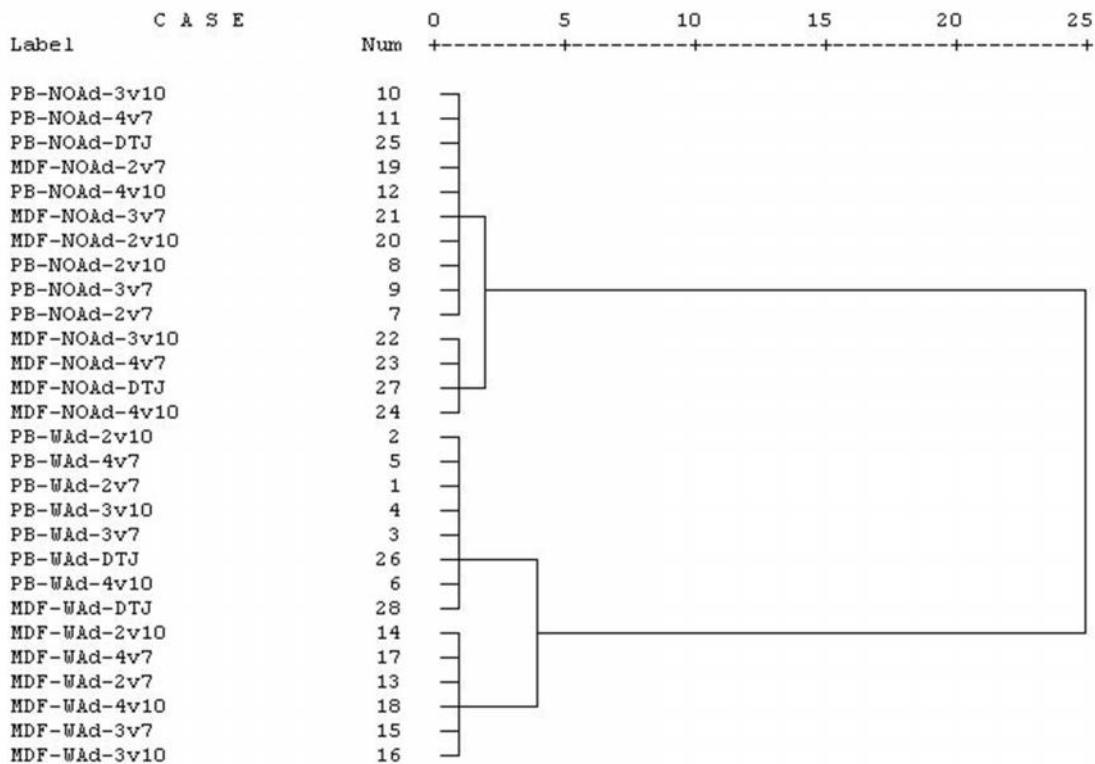
شکل ۷- آنالیز خوشه‌ای ۲۴ تیمار بر مبنای ظرفیت تحمل تنش زیر بارگذاری کششی و فشاری در گوشه درونی و بیرونی اتصالات (MDF = تخته فیبر با دانسیته متوسط، PB = تخته خرده چوب، NOAd = اتصال‌دهنده بدون چسب، WAd = اتصال‌دهنده با چسب، ۳۷، ۲۷ و ۴۷ = تعداد اتصال‌دهنده ۷- شکل، ۷ و ۱۰ = ارتفاع اتصال‌دهنده ۷- شکل، DTJ = اتصال‌دهنده کلید پایون)
