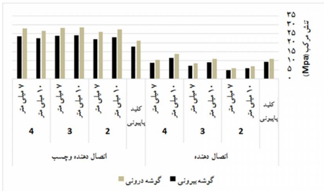
شکل ۶- ظرفیت تحمل تنش زیر بار فشاری در تخته خرده چوب
