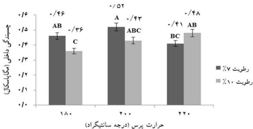
شکل ۷- اثر متقابل رطوبت کیک و حرارت پرس بر چسبندگی داخلی
