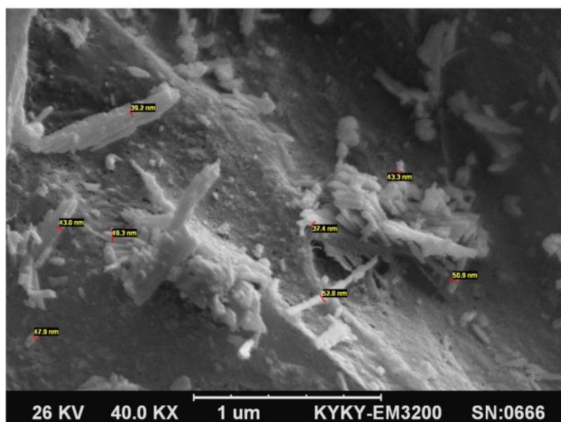
شکل ۱- تصویر SEM نانو سلولز جلبک کلادوفورا
