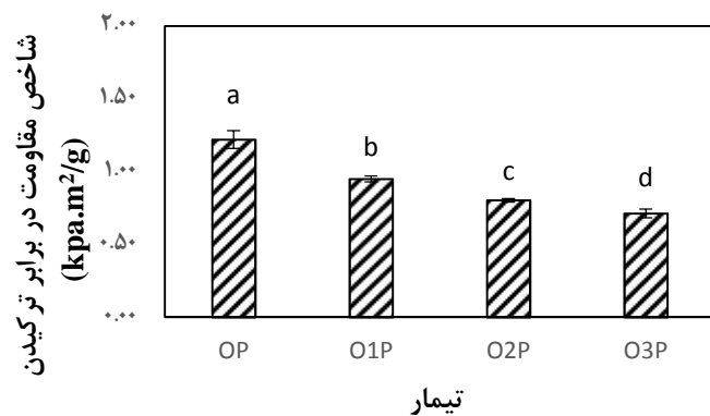
شکل ۵- درصد‌های مختلف پرکننده کربنات کلسیم حاصل از تصفیه آب بر شاخص مقاومت در برابر ترک‌شدن کاغذهای دست‌ساز OCC
