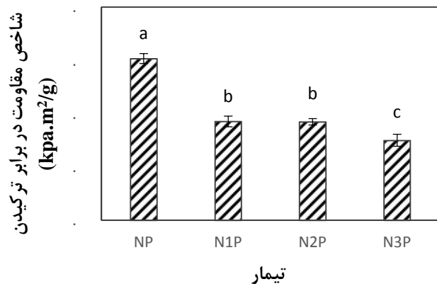
شکل ۶- درصد‌های مختلف پرکننده کربنات کلسیم حاصل از تصفیه آب بر شاخص مقاومت در برابر ترک‌شدن کاغذهای دست‌ساز NSSC
