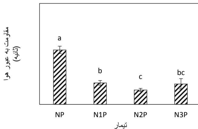
شکل ۲- درصدهای مختلف پرکننده کربنات کلسیم حاصل از تصفیه آب بر شاخص مقاومت به عبور هوا کاغذهای دست ساز NSSC
