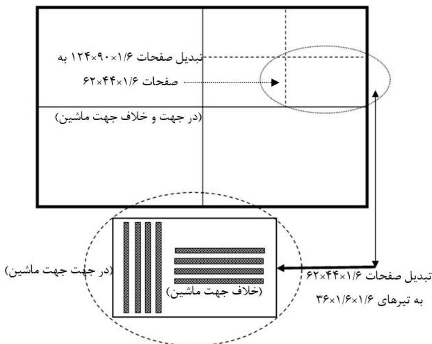
شکل ۳- نحوه تهیه نمونه‌های آزمون از صفحه تا تیر
