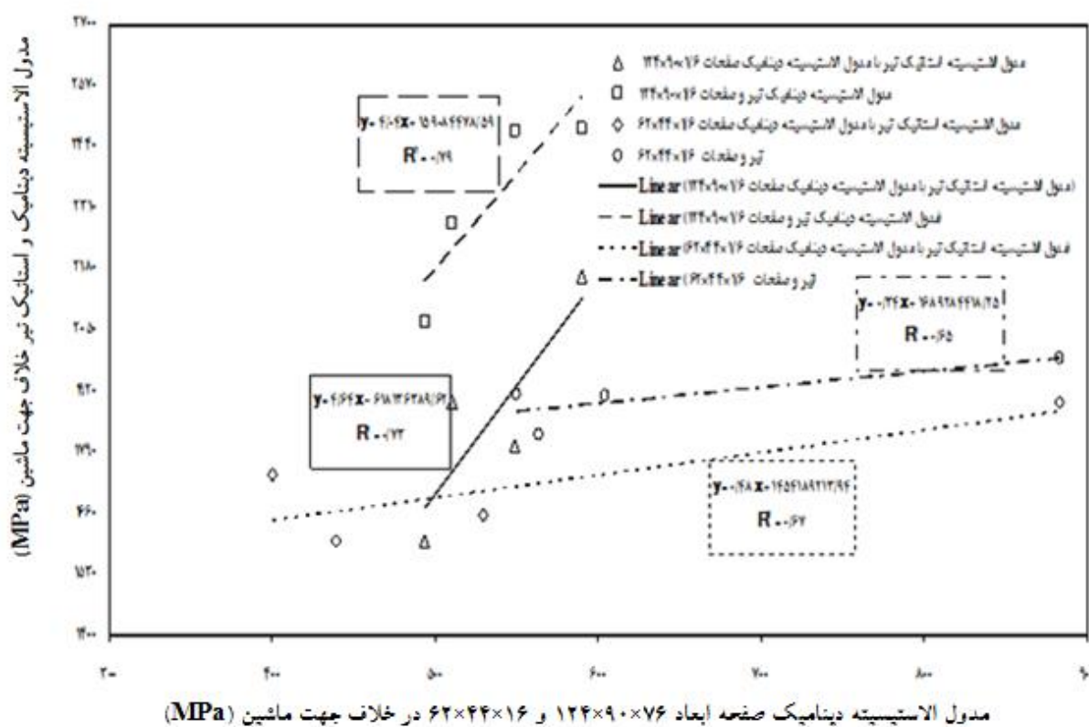
شکل ۵- مقایسه مقادیر مدول الاستیسیته دینامیک صفحات با ابعاد ۱۲۴ \times ۹۰ \times ۱/۶ و ۶۲ \times ۴۴ \times ۱/۶ با مقادیر مدول الاستیسیته استاتیک در جهت خلاف ماشین
