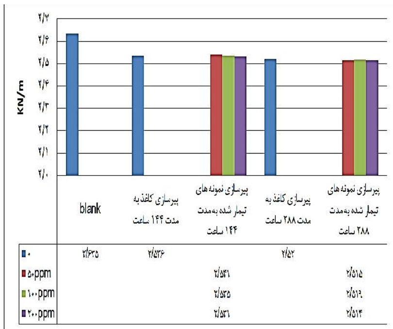
شکل ۶- مقاومت کششی نمونه‌های پیرسازی شده (برحسب KN/m)sh
