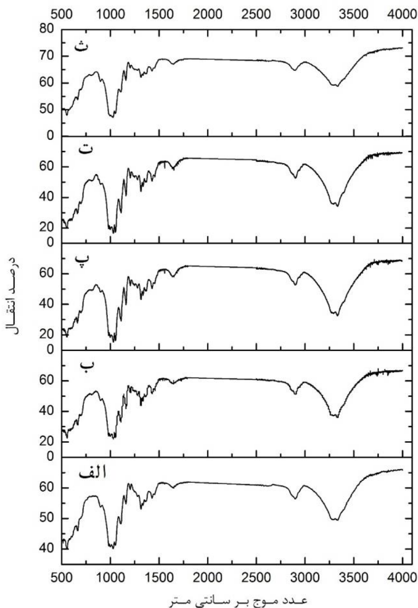
شکل ۷- طیف‌سنجی مادون‌قرمز تبدیل فوریه نمونه‌های الف) آلفا سلولز، ب) CNC0، پ) CNC1، ت) CNC2، ث) CNC3
