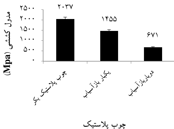
شکل ۴- اثر بازآسیاب بر روی مدول الاستیسیته کششی
