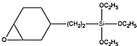
شکل ۲- ساختار ۲- (۴،۳- اپوکسی سیکلوهگزیل) اتیل تری اتوکسی سیلان
