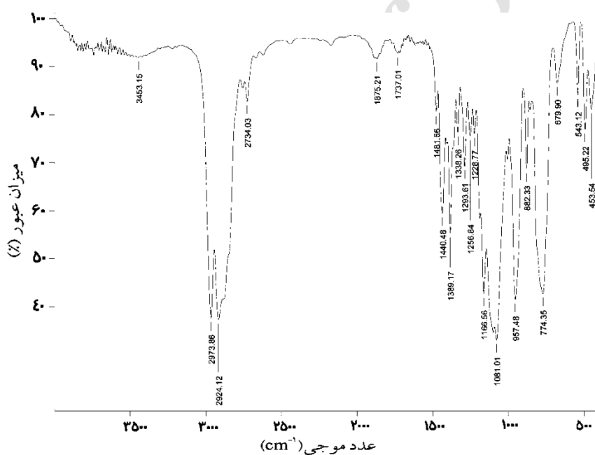
شکل ۴- طیف FTIR از ۲-(۴،۳- اپوکسی سیکلو هگزیل) اتیل تری اتوکسی سیلان
