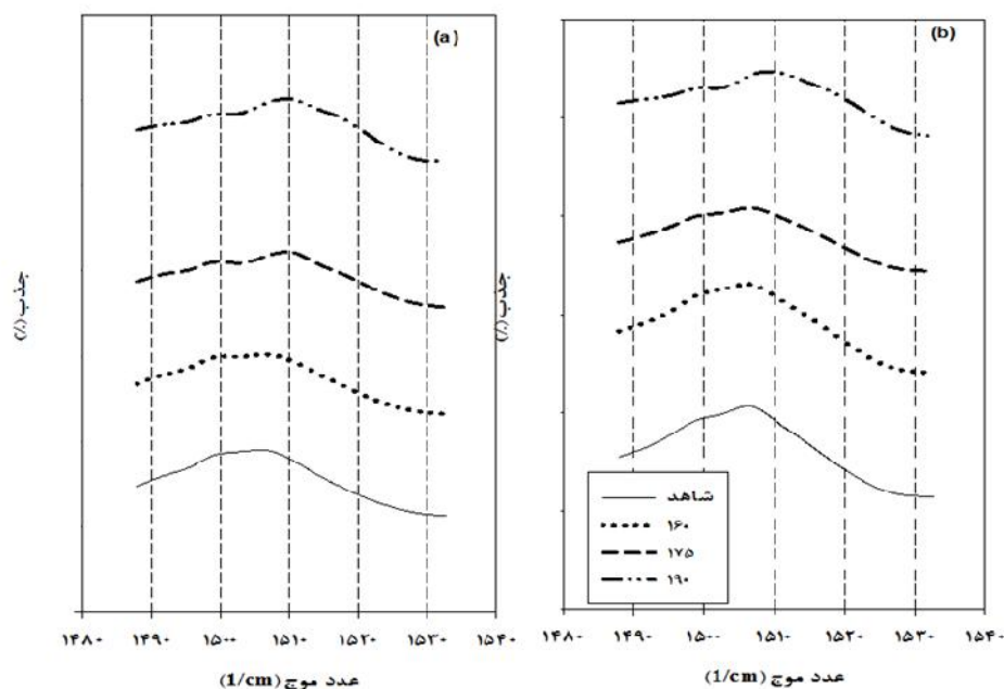
شکل ۳- طیف FTIR گونه‌های راش (a) و افرا (b) در دماهای مختلف اصلاح گرمایی
