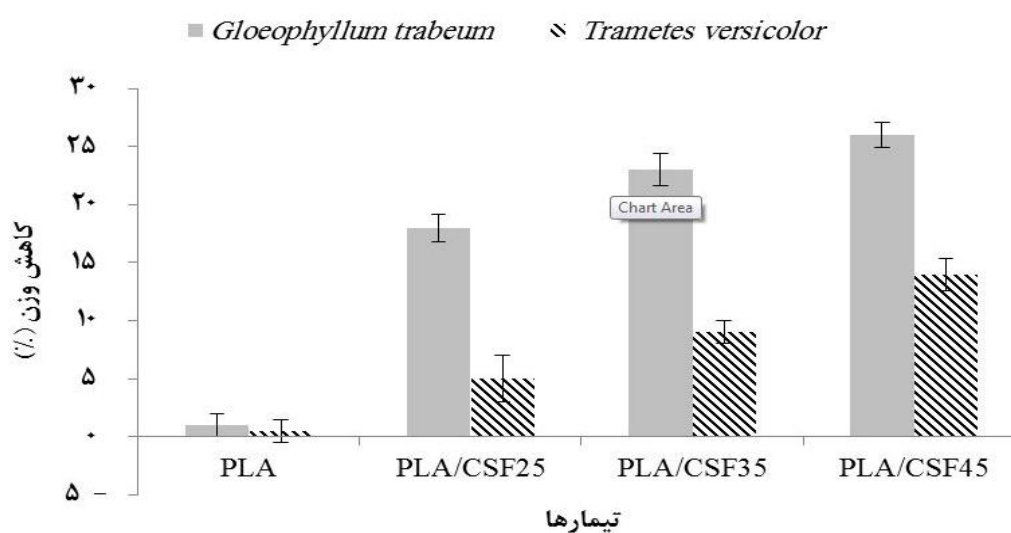
شکل ۳- کاهش وزن چندسازه پلی‌لاکتیک اسید-آرد ساقه کلزا در برابر قارچ‌های عامل پوسیدگی سفید و قهوه‌ای در مدت ۴ ماه
