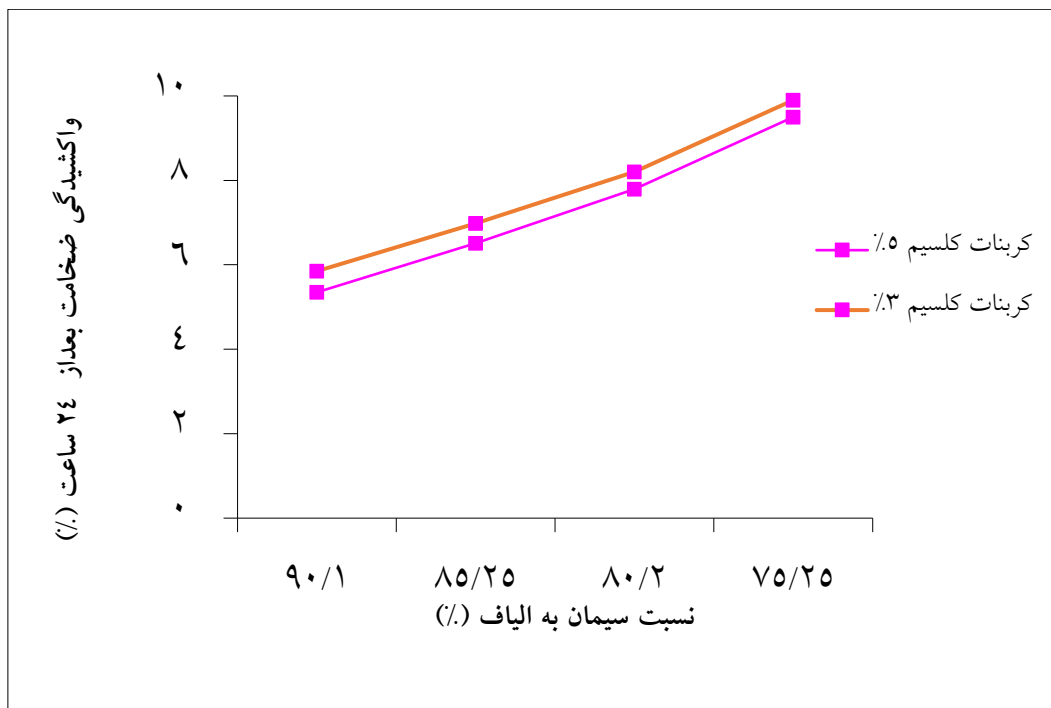
شکل ۵- اثر متقابل نسبت الیاف-سیمان و میزان مواد افزودنی بر واكشیدگی ضخامت بعد از ۲۴ ساعت غوطه‌وری
