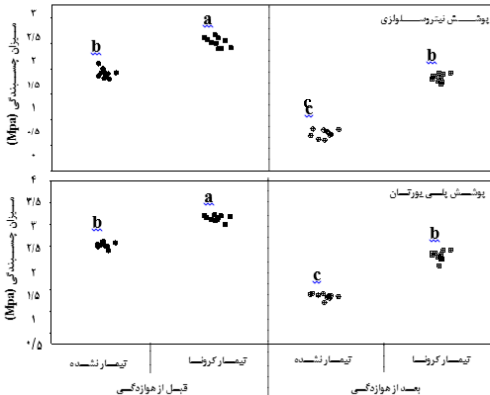
حروف انگلیسی نشان داده شده در تصویر مربوط به گروه بندی دانکن می باشد. شکل ۴- میزان مقاومت به چسبندگی در گونه چوبی راش قبل و بعد از هوازدگی
