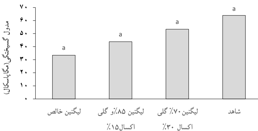
شکل ۶- تأثیر نوع چسب بر مدول گسیختگی تخته لایه
