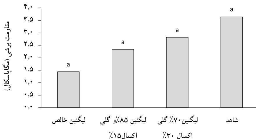
شکل ۴- تأثیر نوع چسب بر مقاومت برشی تخته لایه
