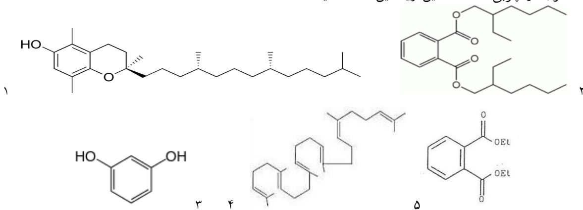
شکل ۵- ساختار بتا-توکوفرول (۱)، بیس (۲- اتیل هگزیل) فتالات (۲)، ریزورسینول (۳)، اسکوتلن (۴) و ۱، ۲- بنزن دی کربوکسیلیک اسید (۵) شناسایی شده در چوب و پوست توت
