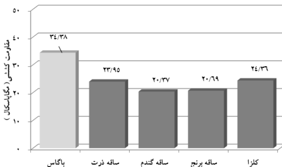
شکل ۷- اثر مستقل مواد لیگنوسلولزی بر مقاومت خمشی نانو چندسازه چوب پلاستیک
