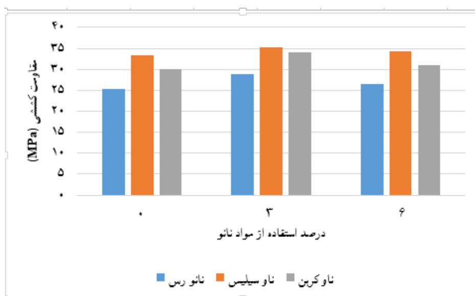
شکل ۸- اثر مستقل درصد مواد نانو بر مقاومت به کشش نانو چندسازه چوب پلاستیک
