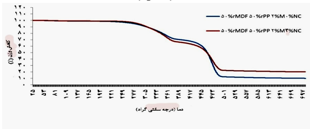
شکل ۳- نمودار مربوط به آزمون گرماسنجی وزنی دو نوع چندسازه با نانورس و بدون آن
