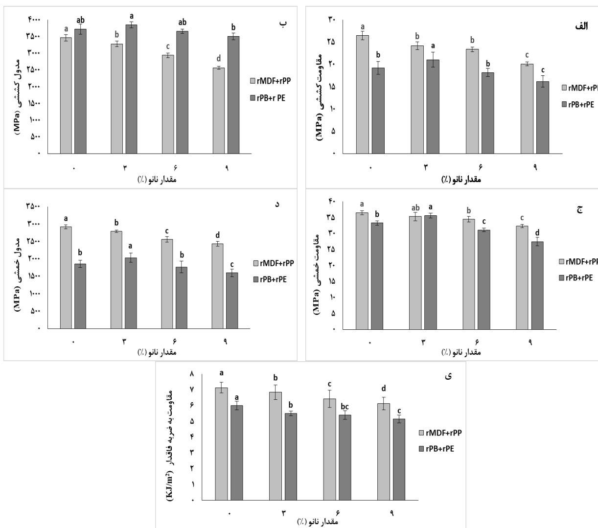
شکل ۱- ویژگی‌های مکانیکی چندسازه‌های ساخته شده با مقادیر مختلف نانورس
