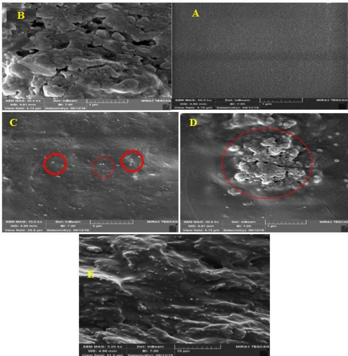
شکل ۳- تصاویر حاصل از میکروسکوپ الکترونی روبشی برای نانو کامپوزیت‌ها و مقطع عرضی فیلم‌های مختلف
