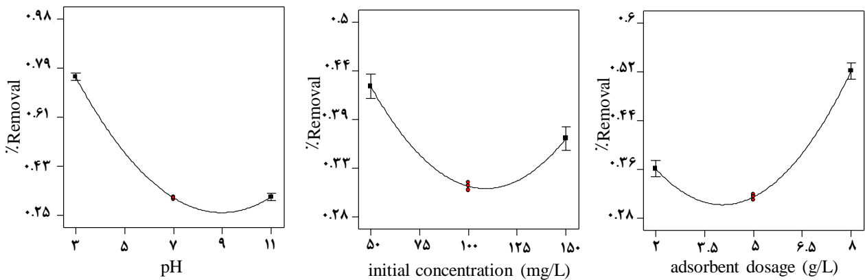
شکل ۴- بررسی تأثیر میانگین عامل‌های اصلی بر روی حذف رنگ اسید سبز ۲۰
