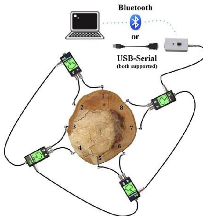
شکل ۲- نحوه اتصال دستگاه توموگرافی امواج تنشی
