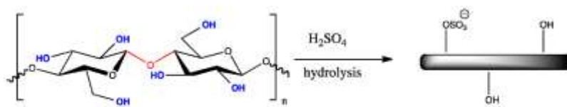
شکل ۱- ساختار میله‌ای نانو کریستال سلولز تولید شده از الیاف سلولزی
