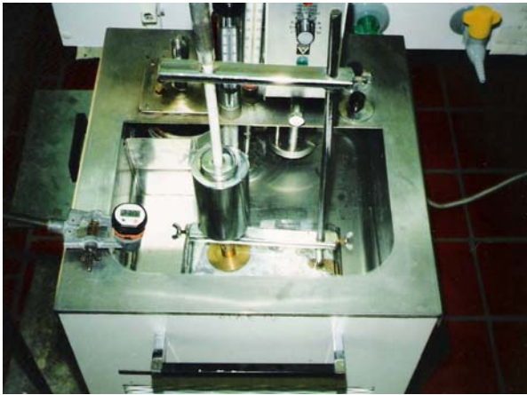
شکل ۲: دستگاه ویژه آزمون سیلان در حمام آب گرم در حین انجام آزمون
