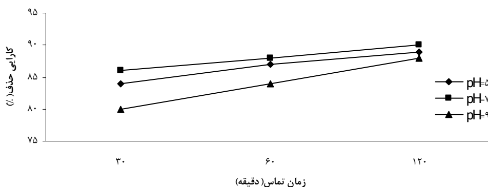
نمودار ۱: بررسی تأثیر تغییرات pH بر کارایی فرآیند مورد مطالعه در حذف فلوراید (محلول فلوراید با غلظت ۲/۴ میلی‌گرم در لیتر و پلی آلومینیوم کلراید با غلظت بیست میلی‌گرم در لیتر)
