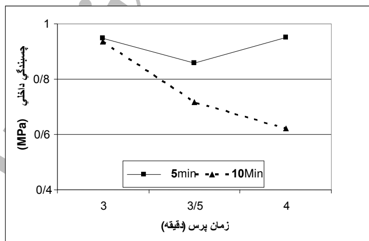
شکل 4 - اثر متقابل زمان بخارزنی و زمان پرس بر چسبندگی داخلی
