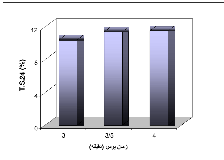
شکل 5 - اثر زمان پرس بر واكشیدگی ضخامت 24 ساعت
