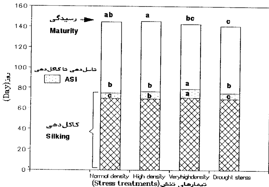
شکل ۱- تأثیر تیمارهای تنش تراکم (۷۰، ۱۰۰ و ۱۴۰ هزار بوته در هکتار) و خشکی بر خصوصیات فنولوژیک ذرت
