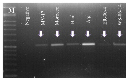
شکل ۳- باندهای تکثیر شده توسط نشانگر Cssfr2 حاصل از الکتروفورز برای تعدادی از ارقام و لاین‌های گندم مورد بررسی. M: مارکر وزنی ۵۰ bp و باندهایی که با پیکان نشان داده شده‌اند، بیانگر آلل Lr34 (۵۲۳ bp) هستند
