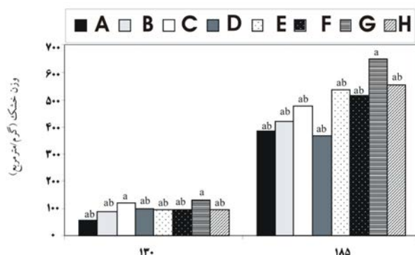
شکل ۳ وزن خشک اندام هوایی چغندرقد در تیمارهای آزمایشی نسبت به شاهد (با علف‌هرز) براساس آزمون دانکن حروف مشابه در هر گیاه نشان‌دهنده عدم اختلاف معنی‌دار در سطح احتمال پنج درصد می‌باشد.
