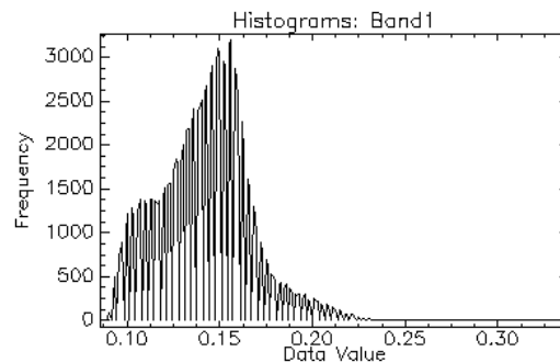
شکل ۳ هیستوگرام باند ۱
