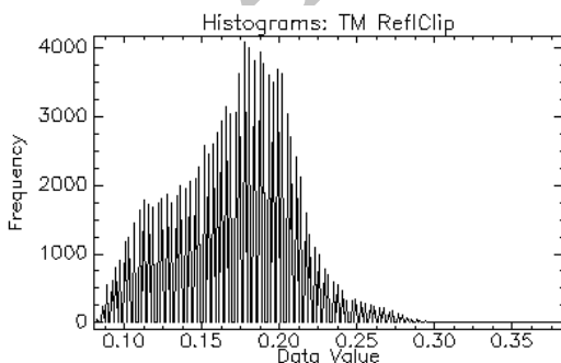
شکل ۴ هیستوگرام باند ۲
