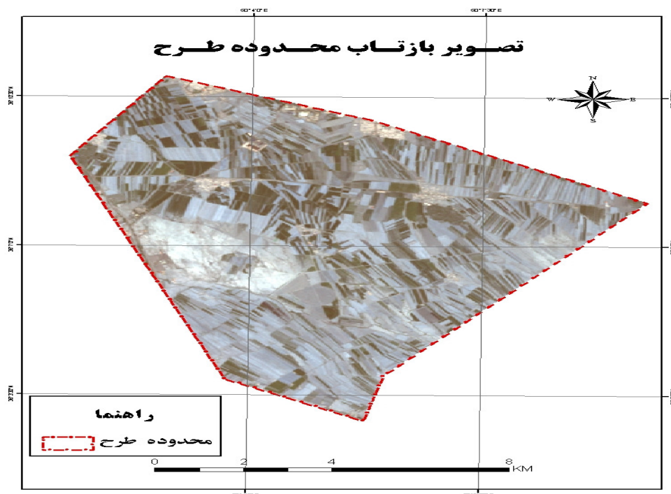
شکل ۲ تصویر بازتاب TM منطقه مورد مطالعه (در ترکیب باندی ۲, ۳, ۴: RGB)
