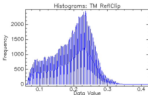
شکل ۵ هیستوگرام باند ۳
