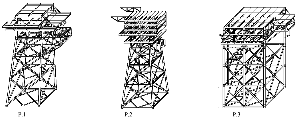
شکل ۴- شکل سه بعدی سکوی مورد استفاده در تحلیل‌ها
