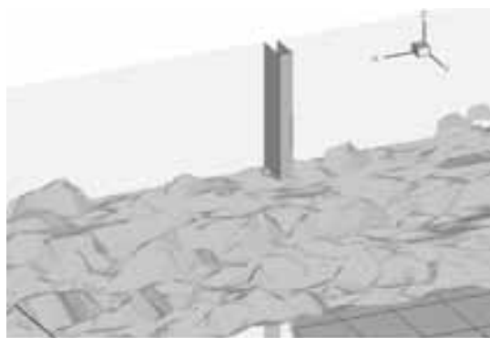
شکل ۴ - نمای سه بعدی سطح آب نزدیک آبشکن با استفاده از شبکه‌های هرمی
