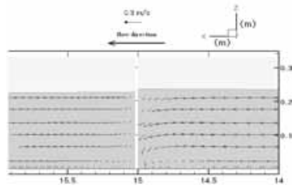
شکل ۲۰ - بردارهای سرعت در صفحه Y=0.1m در کانال ۳۰ متری
