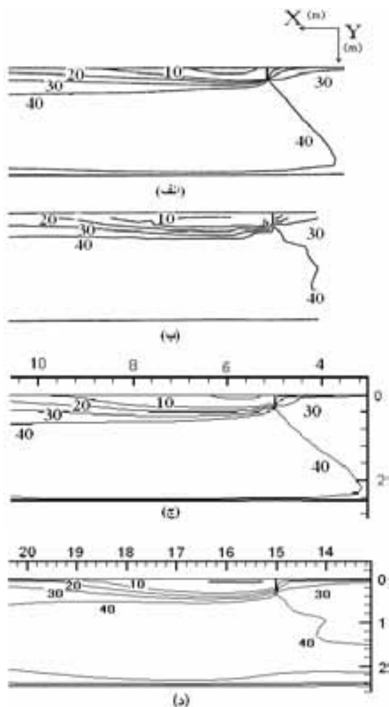
شکل ۱۲- منحنی‌های هم تراز سرعت در تراز ۱۷ cm بالای بستر (الف): نتایج مدل عددی اولیون و دارتوس، (ب): نتایج تجربی، (ج) نتایج مدل سازی با Fluent در کانال ۲۰ متری، (د): نتایج مدل سازی با Fluent در کانال ۳۰ متری
