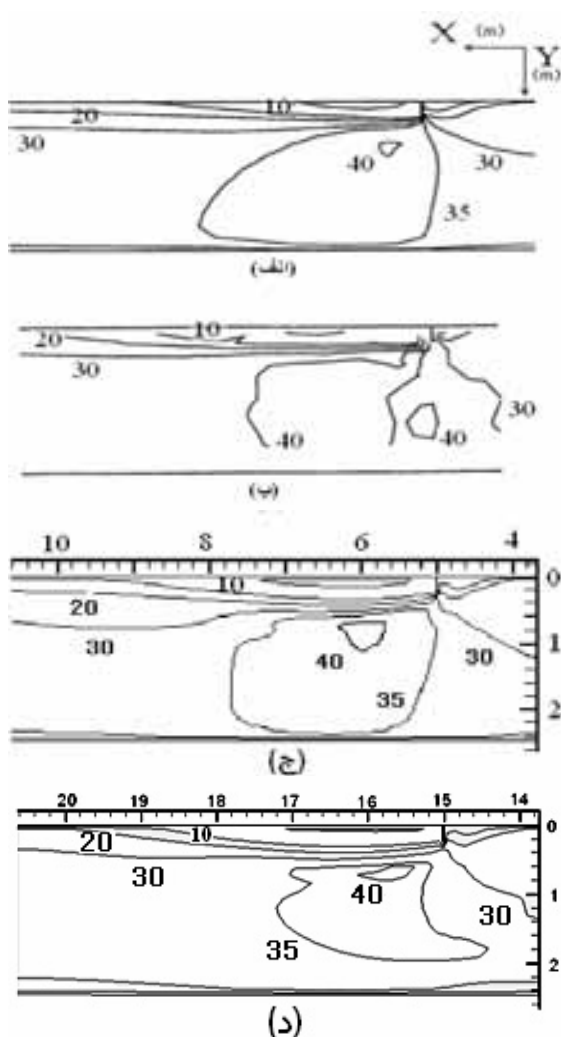
شکل ۱۱- منحنی‌های هم تراز سرعت در تراز ۵ cm بالای بستر (الف): نتایج مدل عددی اولیون و دارتوس، (ب): نتایج تجربی هلنز، (ج): مدل سازی با Fluent در کانال ۲۰ متری، (د): مدل سازی با Fluent در کانال ۳۰ متری
