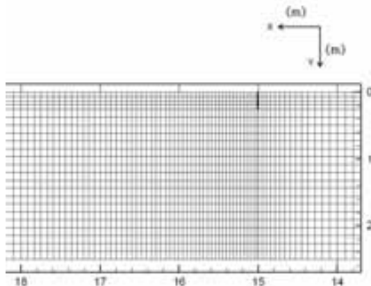
شکل ۳ - شبکه بندی کانال در پلان در کانال ۳۰ متری
