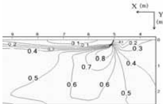
شکل ۲۰ - منحنی های هم تراز تنش برشی در تراز بستر (pa)
