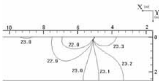
شکل ۱۸ - منحنی های هم تراز سطح آزاد آب
