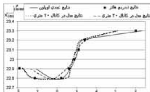
شکل ۸ - مقایسه پروفیل سطح آزاد در صفحه Y=0.8m
