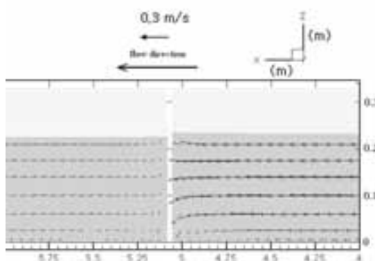
شکل ۱۹ - بردارهای سرعت در صفحه Y=0.1m
