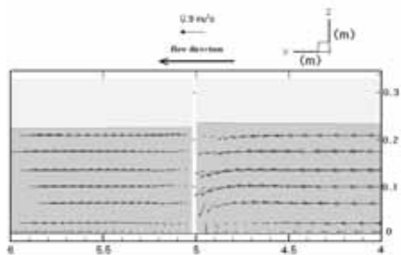
شکل ۲۱ - بردارهای سرعت در صفحه Y=0.1m در کانال ۲۰ متری
