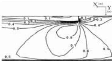
شکل ۱۶: نتایج عددی اویلون و دارتوس
