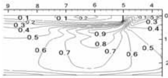
شکل ۱۷: تنش برشی در کانال ۲۰ متری
