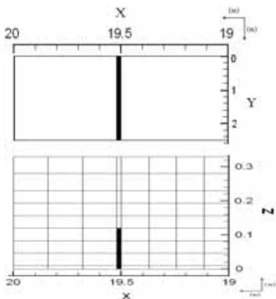
شکل ۵ - پلان سرریز انتهای کانال و نمای شبکه بندی در عمق
