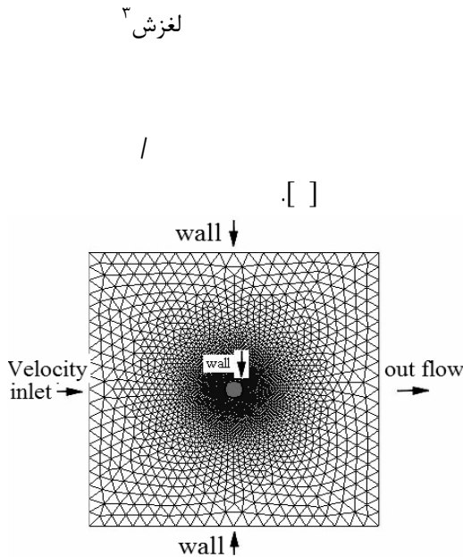
شکل ۷- مدل هندسی محیط و شبکه بندی آن.
