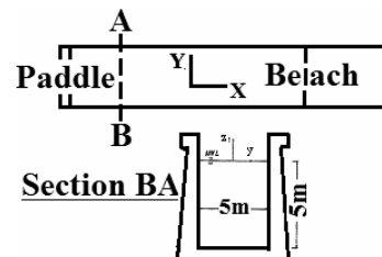
شکل ۳- طرح شماتیک کانال موج دلتا
