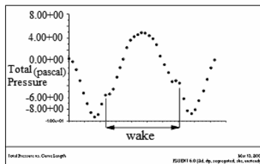
شکل ۹- توزیع فشار حول نمونه و تعیین موقعیت ناحیه دنباله
