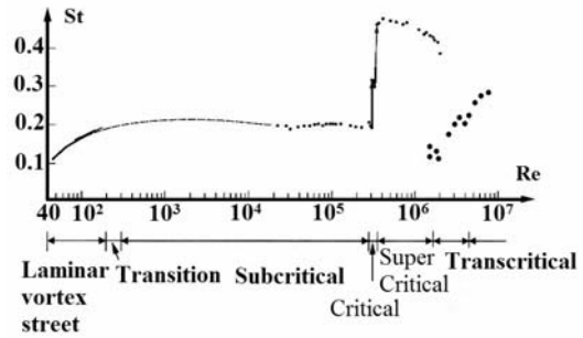
شکل ۲- مقدار عدد استروهل برای یک استوانه
