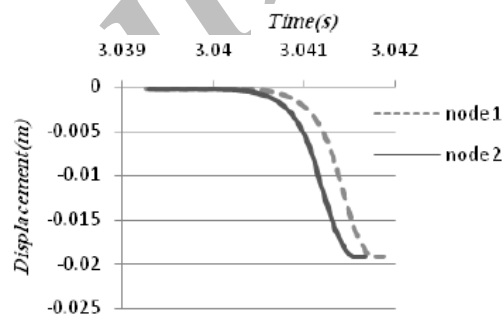
شکل ۷- نمودار تاریخچه زمانی جابجایی برای دو گره انتخابی روی مدل
