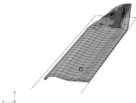
شکل ۹- تغییر شکل ناشی از انتشار کماتش دینامیکی
