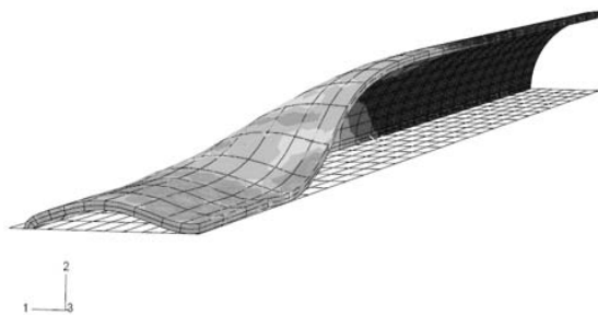
شکل ۶- انتشار کمانش شبه استاتیکی
