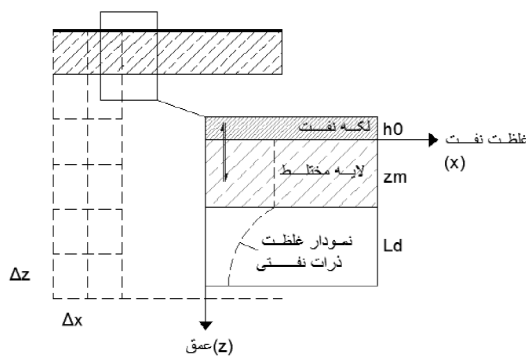
شکل ۱- لایه نفتی و لایه اختلاط آب و نفت و همچنین شبکه محاسباتی مربوطه [۷]
