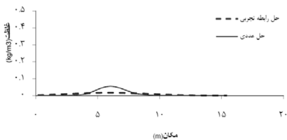
شکل ۱۲ - نمودار تغییرات غلظت در مکان (۵ و x) در T=40 s
