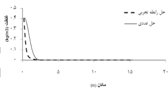
شکل ۱۰ - نمودار تغییرات غلظت در مکان (۵ و x) در T=2.5 s [مبدأ مختصات بر روی نقطه رها شده لکه نفتی قرار دارد]
