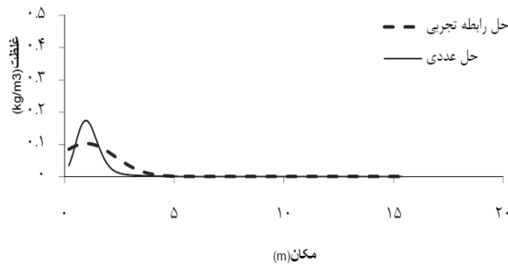
شکل ۱۱ - نمودار تغییرات غلظت در مکان (۵ و x) در T=10 s
