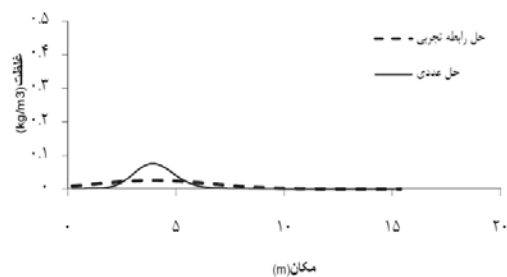
شکل ۱۳ - نمودار تغییرات غلظت در مکان (۵ و x) در T=70 s
