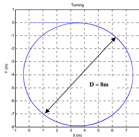
شکل ۱۱- تست دایره چرخش SUT-2 با زاویه باله ۱۵ درجه و دور موتور ۱۰۰۰ rpm
