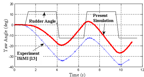
شکل ۷- مقایسه زاویه چرخش در تست تجربی و شبیه‌سازی کامپیوتری
