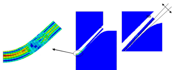
شکل ۱۴- شبیه‌سازی برگشت فنری با شعاع قالب ۳ میلی متر
