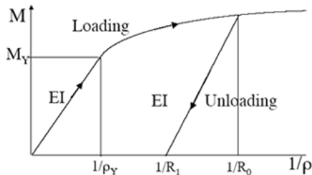
شکل ۲- منحنی گشتاور خمشی- انحناء
