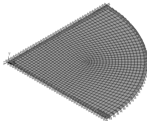
شکل ۶- شرایط مرزی در ورق تحت شکل‌دهی
