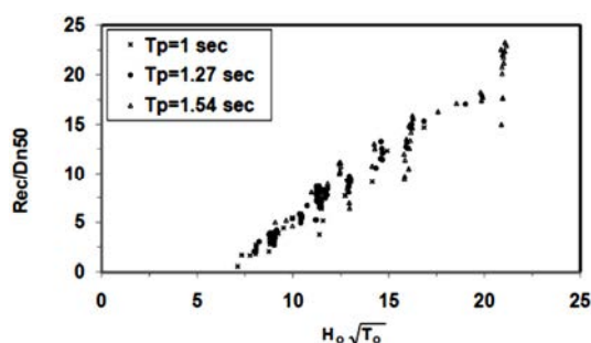
شکل ۱۰ - نمودار تغییرات عرض فرسایش یافته بدون بعد سکو بر حسب پارامتر H_0 \sqrt{T_0}
