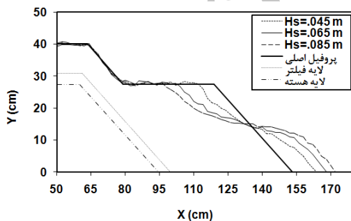
شکل ۶- مقایسه نیم رخ تغییر شکل یافته تحت اثر ارتفاع امواج (قطر سنگداده ها ۱۷٪ متر، پریود اوجی موج ۱/۲۷ ثانیه و عرض سکو ۴۰ سانتی متر)
