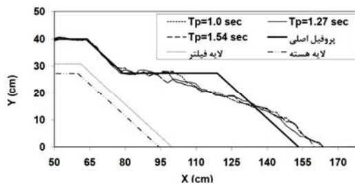
شکل ۷ - نیمرخ تغییر شکل یافته تحت اثر پریود امواج (قطر سنگدانه ها 0.21 متر و ارتفاع موج 1.0/55 سانتی-متر)
