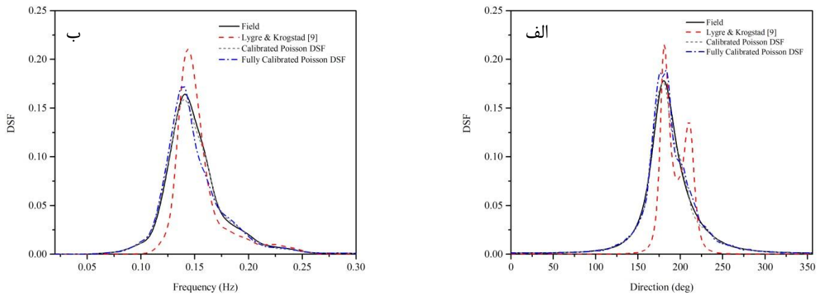
شکل ۱۰. نمای دو بعدی عملکرد توزیع های جهتی استاندارد و کالیبره شده و کاملاً کالیبره شده لیره و کروستاد در مقایسه با میدانی (رخداد از سمت غرب (\theta_0 = 180^\circ) مورخه ۲۰۱۰/۱۲/۱۳) الف: در فرکانس غالب ب: در جهت رخداد موج پریود پیک سمت غرب مورخه ۲۰۱۰/۱۲/۱۳) a: در فرکانس غالب d: در جهت رخداد موج پریود پیک
