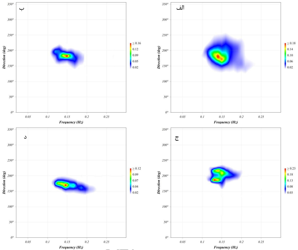
شکل ۵- عملکرد توزیع‌های جهتی استاندارد در مقایسه با توزیع جهتی میدانی "رخداد از سمت غرب" ( \theta_0 = 180^\circ ) مورخه ۲۰۱۰/۱۲/۱۳ "الف: توزیع جهتی میدانی، ب: توزیع جهتی میتسوایسو و همکاران [۶] ج: لیبره و کروستاد [۹] د: دونلن و همکاران [۹]
