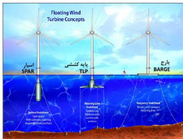
شکل ۱- انواع فونداسیون توربین‌های بادی فراساحلی [۷]
