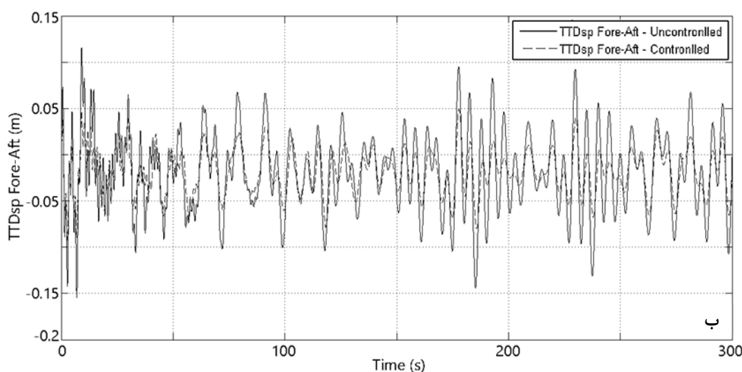
شکل ۳ - پاسخ تاریخچه زمانی جابجایی بالای توربین در دو حالت کنترل شده و کنترل نشده در راستای فور-آفتر (الف): سرعت باد ۱۰ متر بر ثانیه، (ب): سرعت باد ۱۸ متر بر ثانیه
