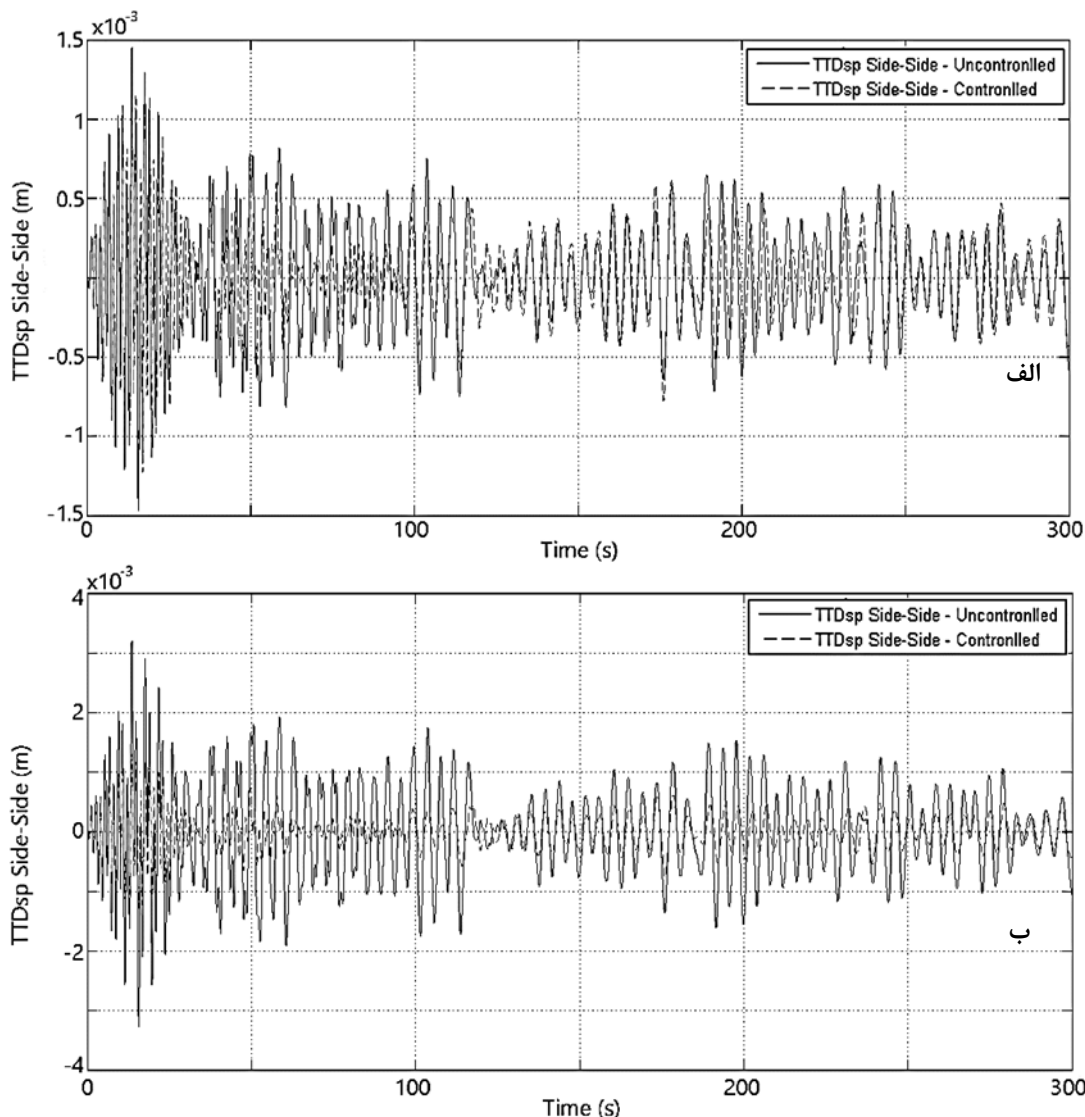
شکل ۵- پاسخ تاریخیچه زمانی جابجایی بالای توربین در دو حالت کنترل شده و کنترل نشده در راستای سایید-ساید (الف): سرعت باد ۱۰ متر بر ثانیه، (ب): سرعت باد ۱۸ متر بر ثانیه
