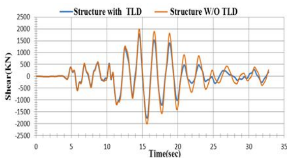
شکل ۱۲- تاریخچه زمانی برش پایه سکو برای حالت‌های با و بدون TLD تحت زلزله‌های:
