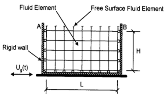
شکل ۶- تصویر شماتیک مدل اجزای محدود دو بعدی مخزن حاوی سیال
