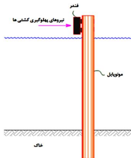
شکل ۱ - شکل مونوپایل به عنوان دولفین پهلوگیری تحت بار جانبی
