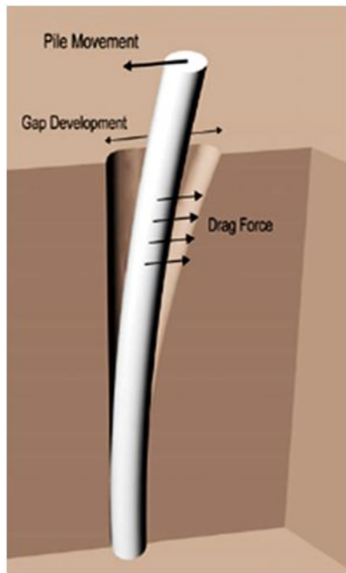
شکل ۲۱- پاسخ خاک و شمع در هنگام باربرداری [۱۶]
