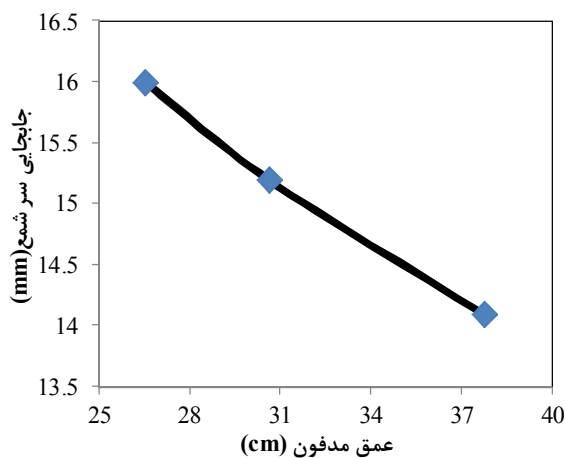
شکل ۱۶ - نمودار اثر عمق مدفون بر جابجایی در سر شمع برای ۳ آزمایش اول
