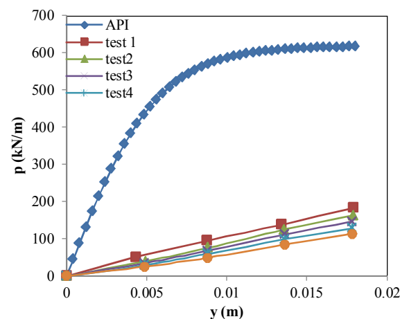
شکل ۲۴ - مقایسه منحنی p-y آزمایش‌ها و API در عمق Z=3D
