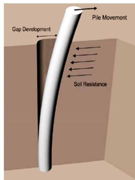
شکل ۲۰- پاسخ خاک و شمع در هنگام بارگذاری [۱۶]
