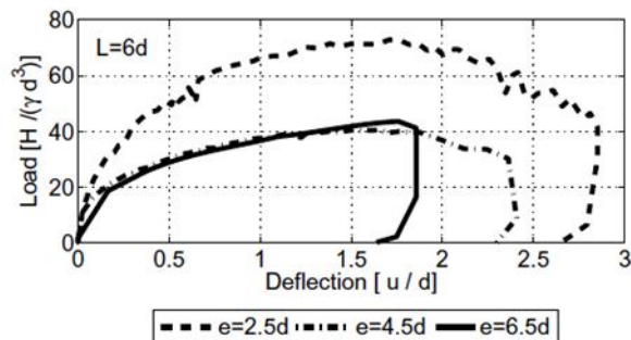
شکل ۷- نمودارهای نیرو- تغییر مکان سرشمع در طول آزاد و عمق مدفون‌های متفاوت [۱۴]
