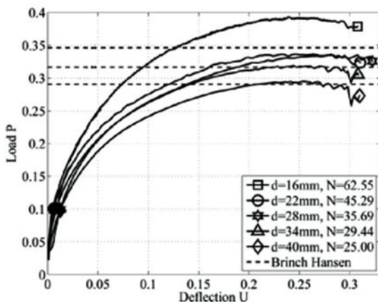
شکل ۵- منحنی‌های نیرو - تغییر مکان سر شمع با شتاب متفاوت [۱۳]
