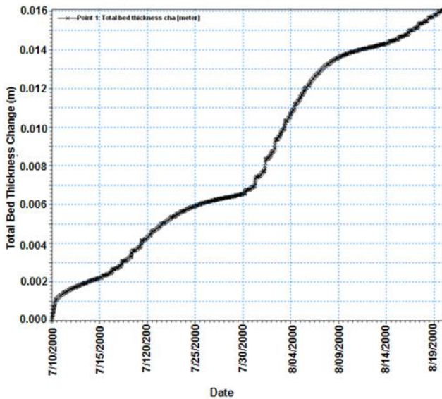
شکل ۲۰- رسوب گذاری در محل لنگرگاه اسکله خدمات بندری در مدت ۴۰ روز
