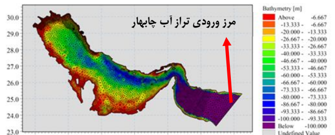
شکل ۱۲- چگونگی شبکه‌بندی در دامنه محاسباتی مدل کلی جریان
