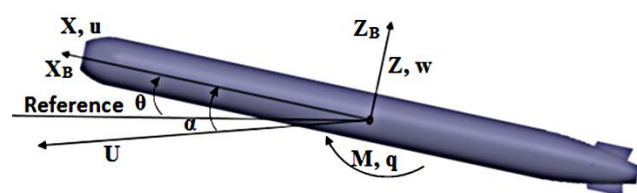
شکل ۱- سیستم مختصات
