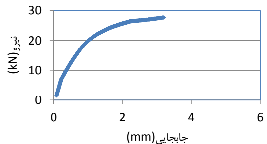
شکل ۲۶- نمودار تست کشش نمونه W۳.
