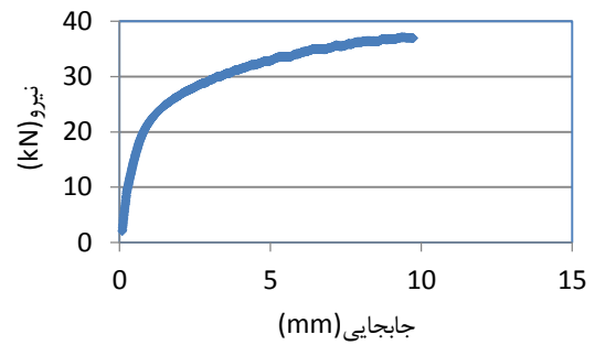
شکل ۲۴- نمودار تست کشش نمونه W۱.
