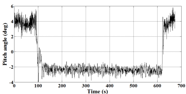
شکل ۷- تخمین زاویه‌ی فراز در تست اول
