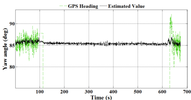
شکل ۸- تخمین زاویه‌ی سمت در تست اول
