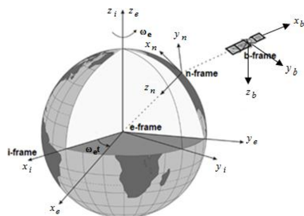
شکل ۲- دستگاه‌های مختصات مختلف در ناوبری اینرسی [۱۶]
