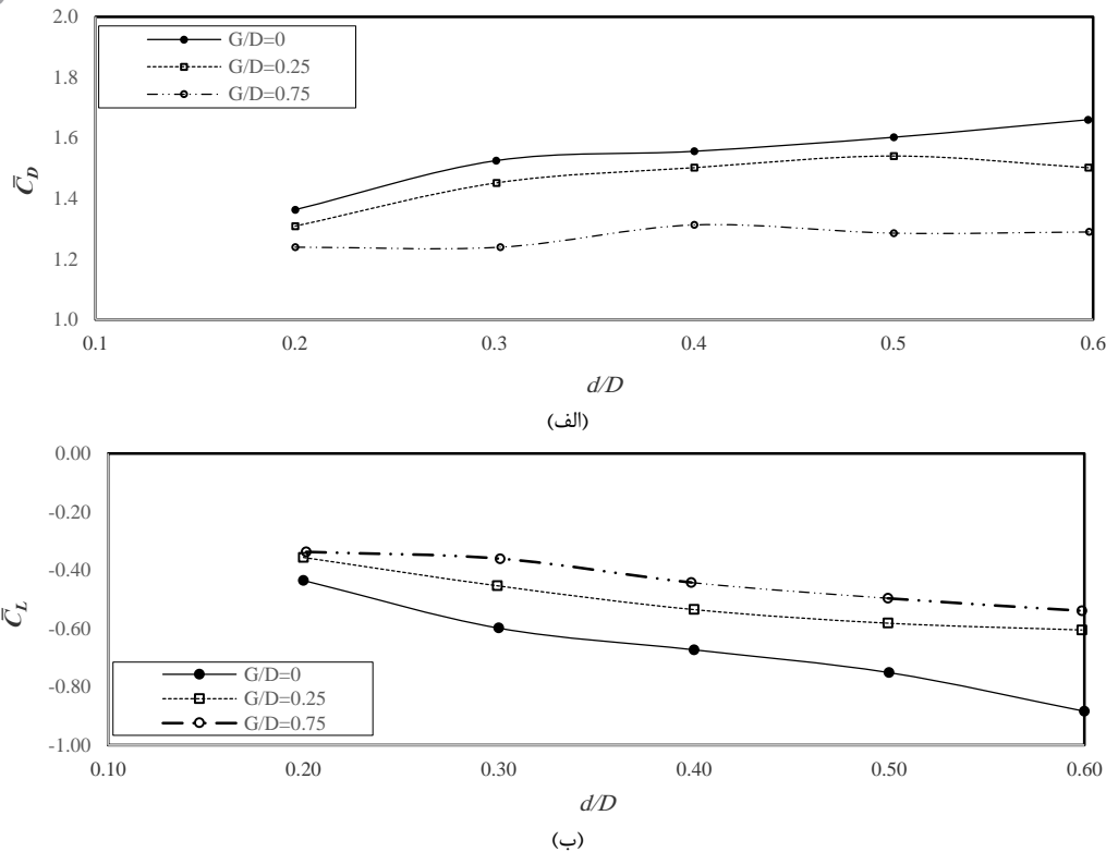
شکل ۵- اثر قطر نسبی بر تغییرات مقدار (الف) ضریب دراگ و (ب) ضریب لیفت وارده بر استوانه اصلی ( Re = 2/\Delta \times 10^4 )
