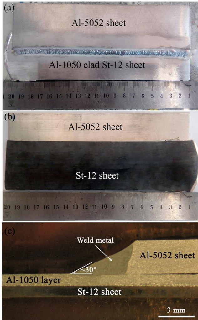
شکل ۷- ظاهر جوش: (a) نمای جلو و (b) نمای پشت جوش و (c) ماکروساختار مقطع عرضی جوش با حرارت ورودی 290 \text{ J mm}^{-1}
