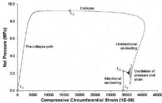
شکل ۳- نمودار تنش کرنش [۷]
