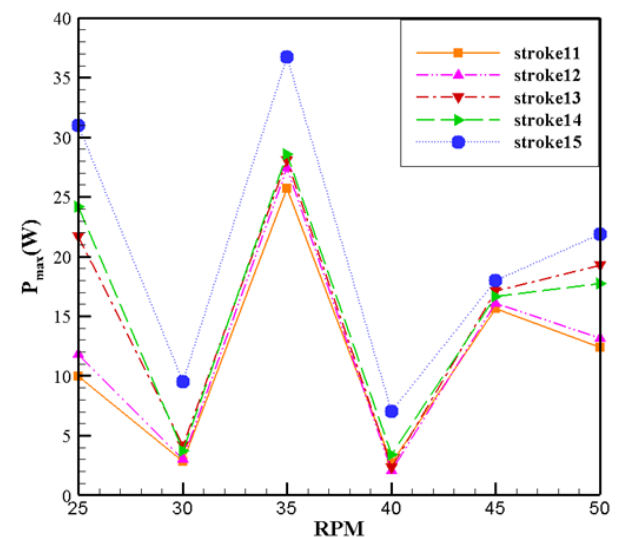
شکل ۱۰: نمودار ماکزیمم توان تولیدی بر حسب دور موتور برای ۱۵ دامنه موج مختلف
