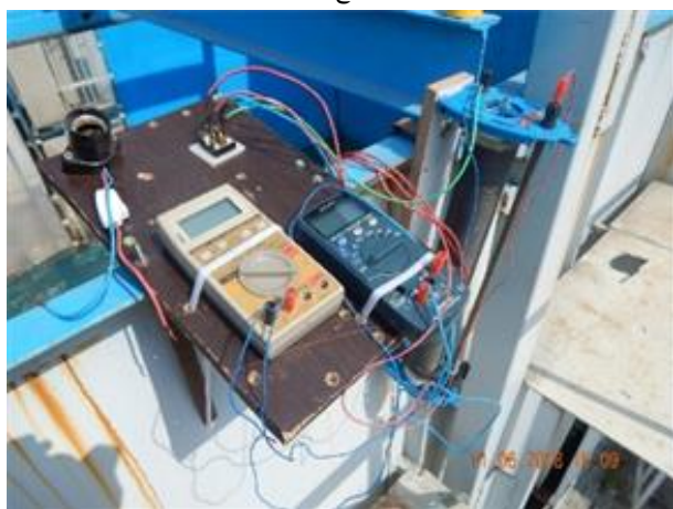
شکل ۵: الف) مجموعه کامل مبدل انرژی موج مستقر در استخر موج (ب) مجموعه چرخ دنده، چرخ طیار و ژنراتور (ج) مجموعه رنوستا و مولتی متر-ها برای ثبت ولتاژ و جریان تولیدی توسط سامانه
