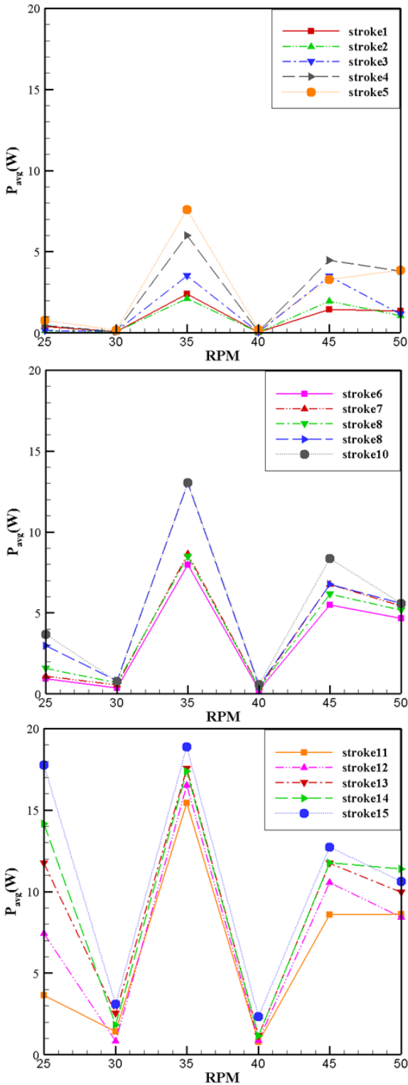
شکل ۷: نمودار متوسط توان تولیدی بر حسب دور موتور برای ۱۵ دامنه موج مختلف
